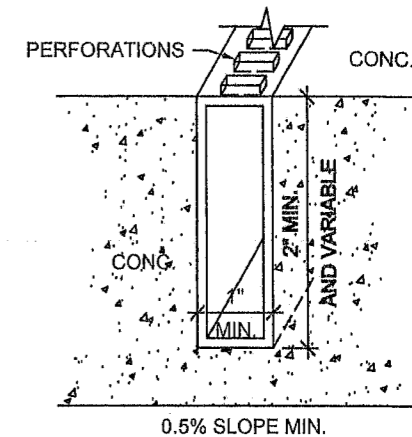
DECK DRAIN DETAIL N.T.S.
